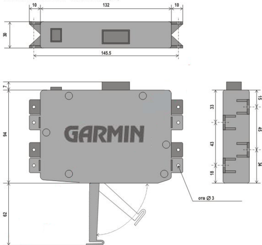
Рис. 22. Габаритные размеры GVN-51.
