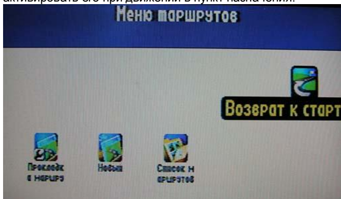
Рис. 15. Меню маршрутов.
