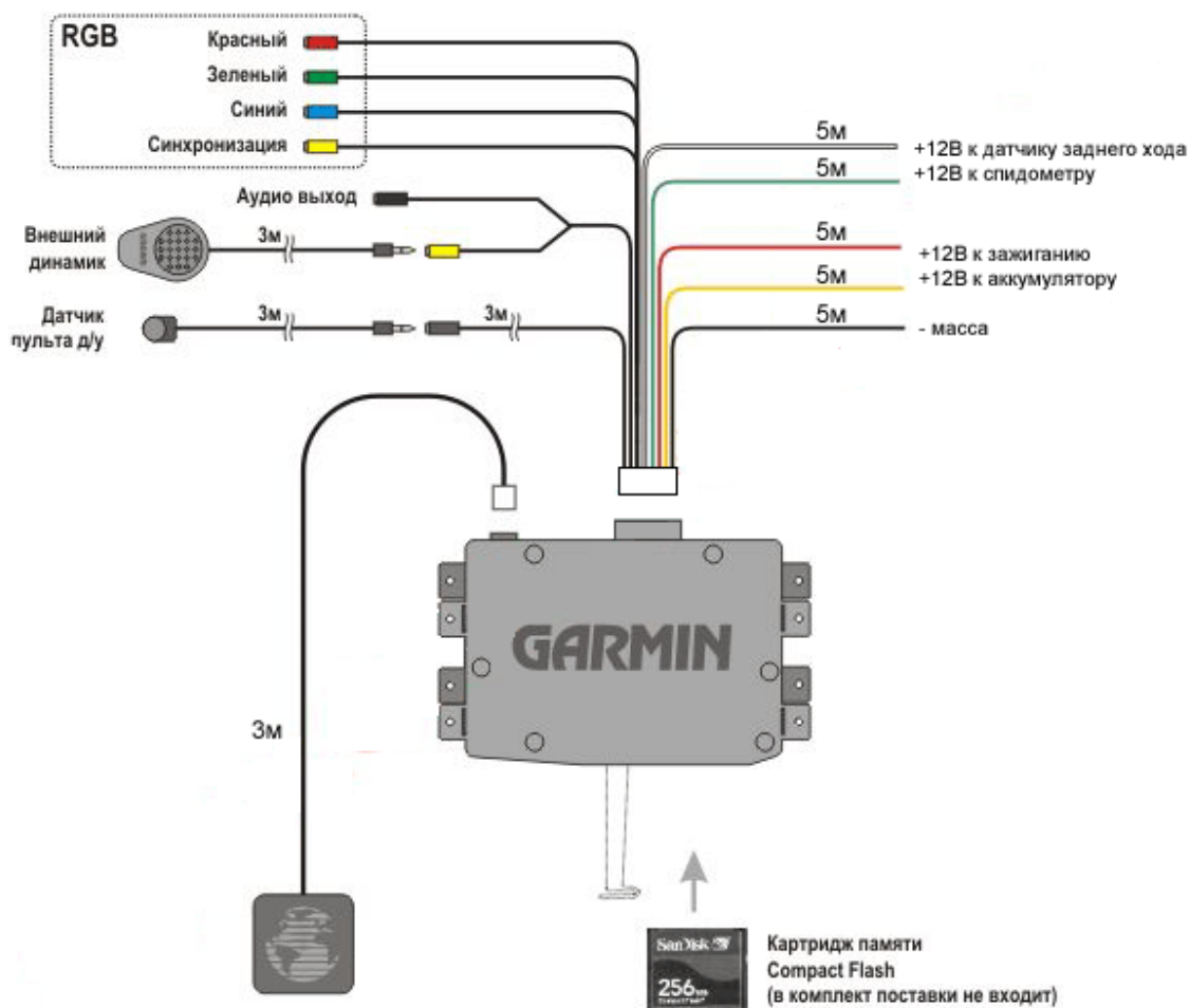
Рис. 20. Схема подключения. Вариант с выходом RGB.
