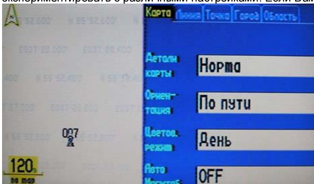
Рис. 13. Настройка карты.
